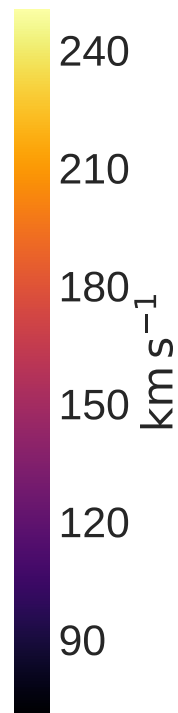
8485-1901 stellar_sigma
