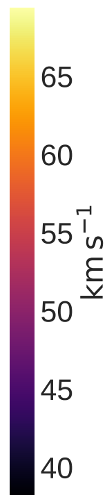
7443-12701 stellar_sigma
